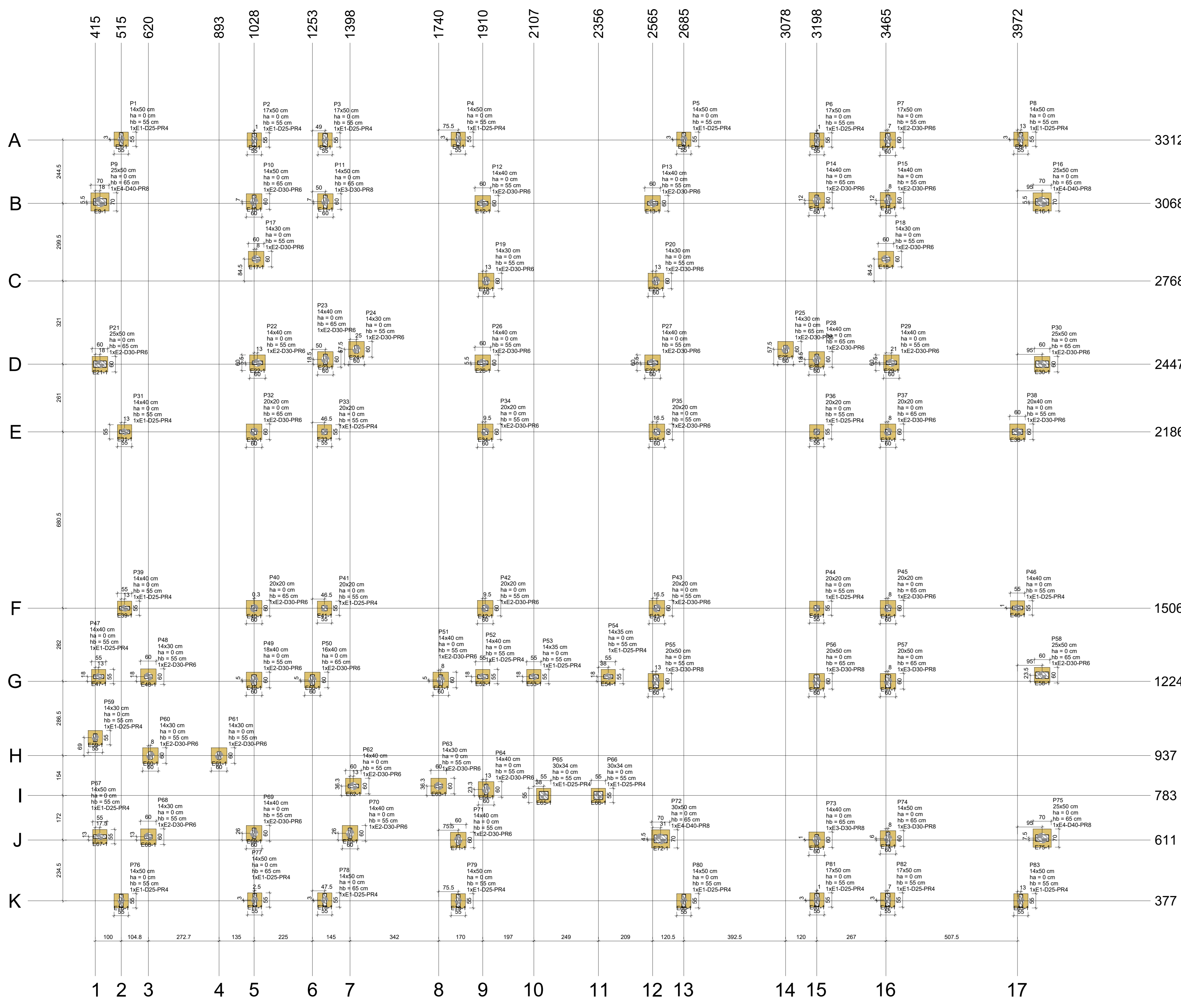
Planta de locação das estacas escala 1:75
