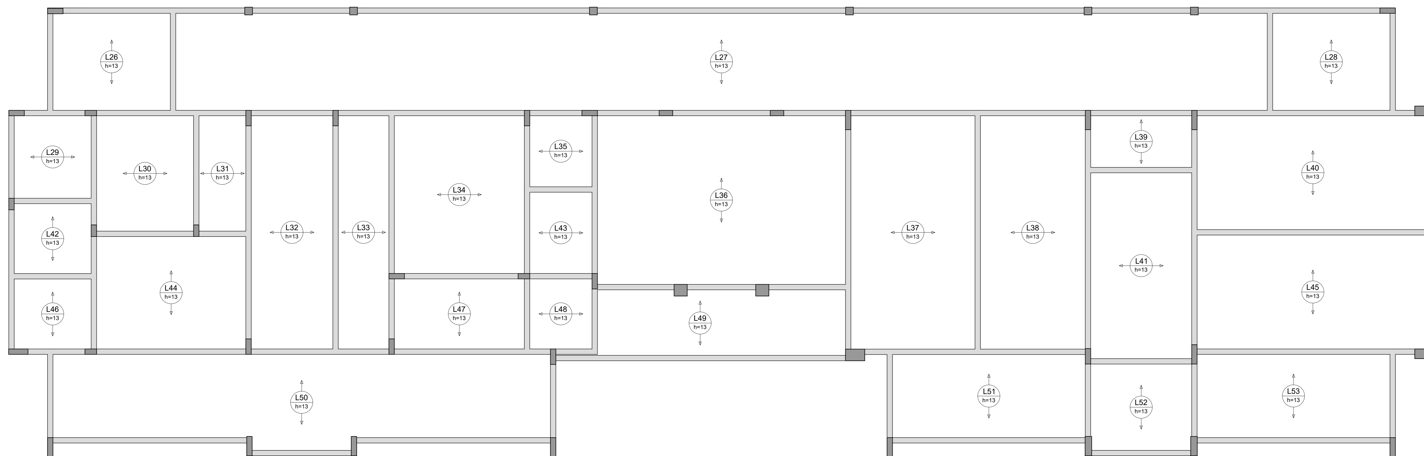
Armação positiva das lajes do pavimento COBERTURA (Eixo Y) escala 1:50
