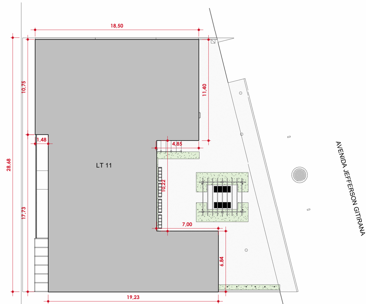
LOCAÇÃO ESC:1 : 250
