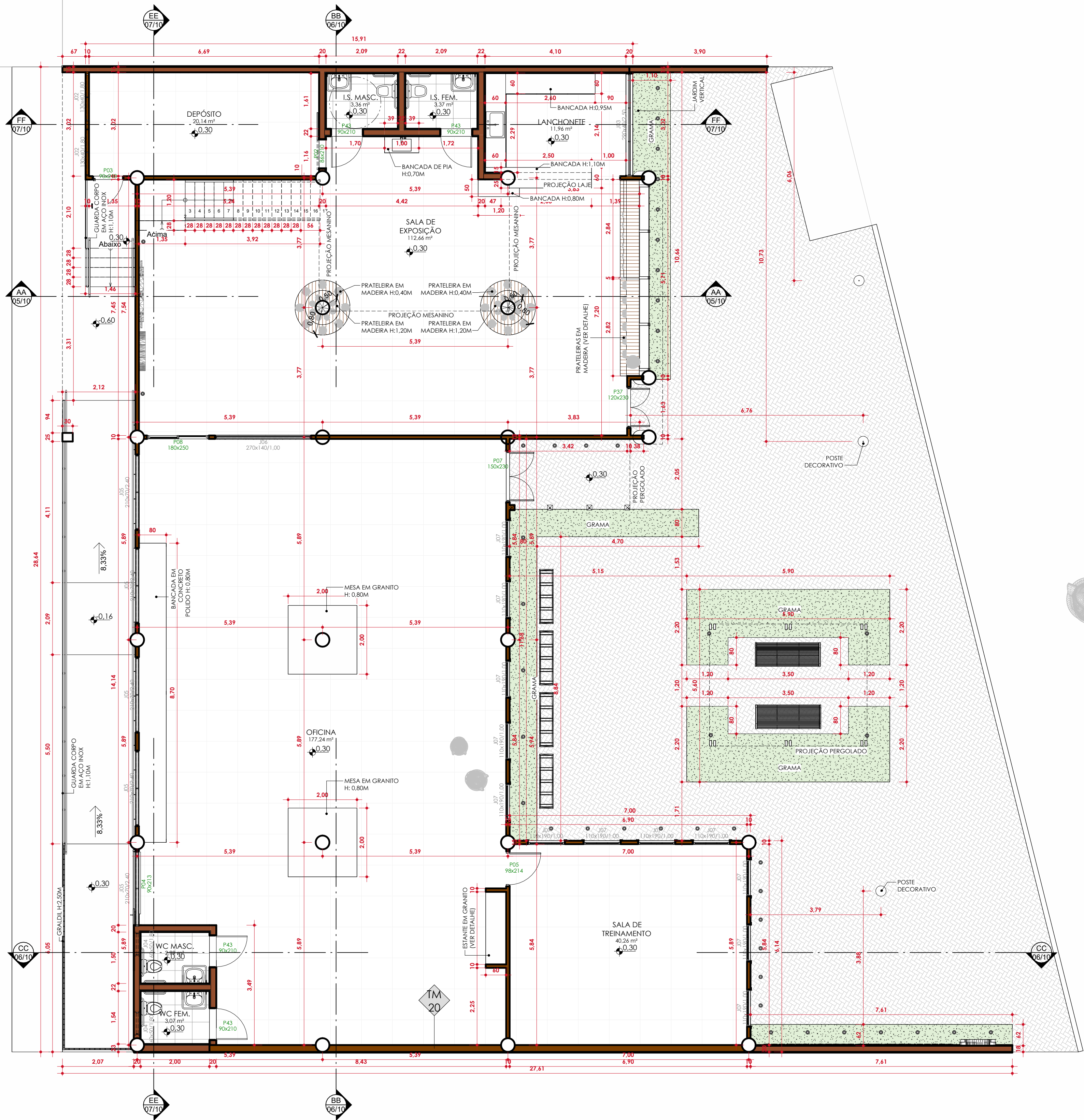
TÉRREO ESC:1 : 75
