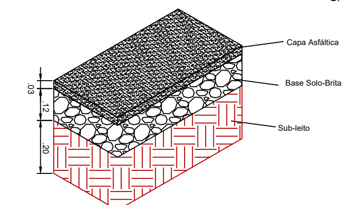
CAMADAS PAVIMENTO S/ ESCALA
