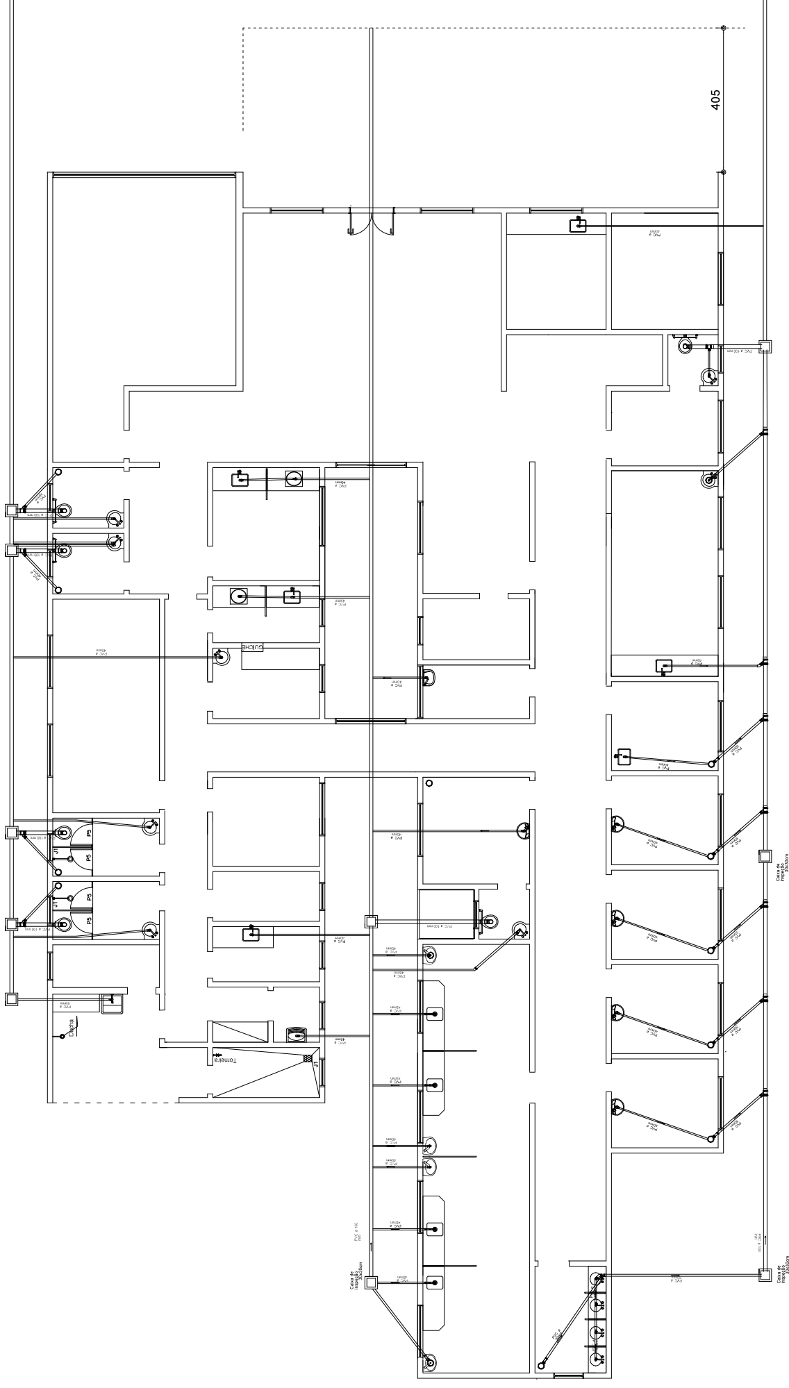
PLANTA DE ESGOTO SANITÁRIO esc 1:100
