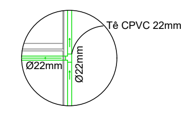
06 DETALHE 3 ESCALA 1:20
