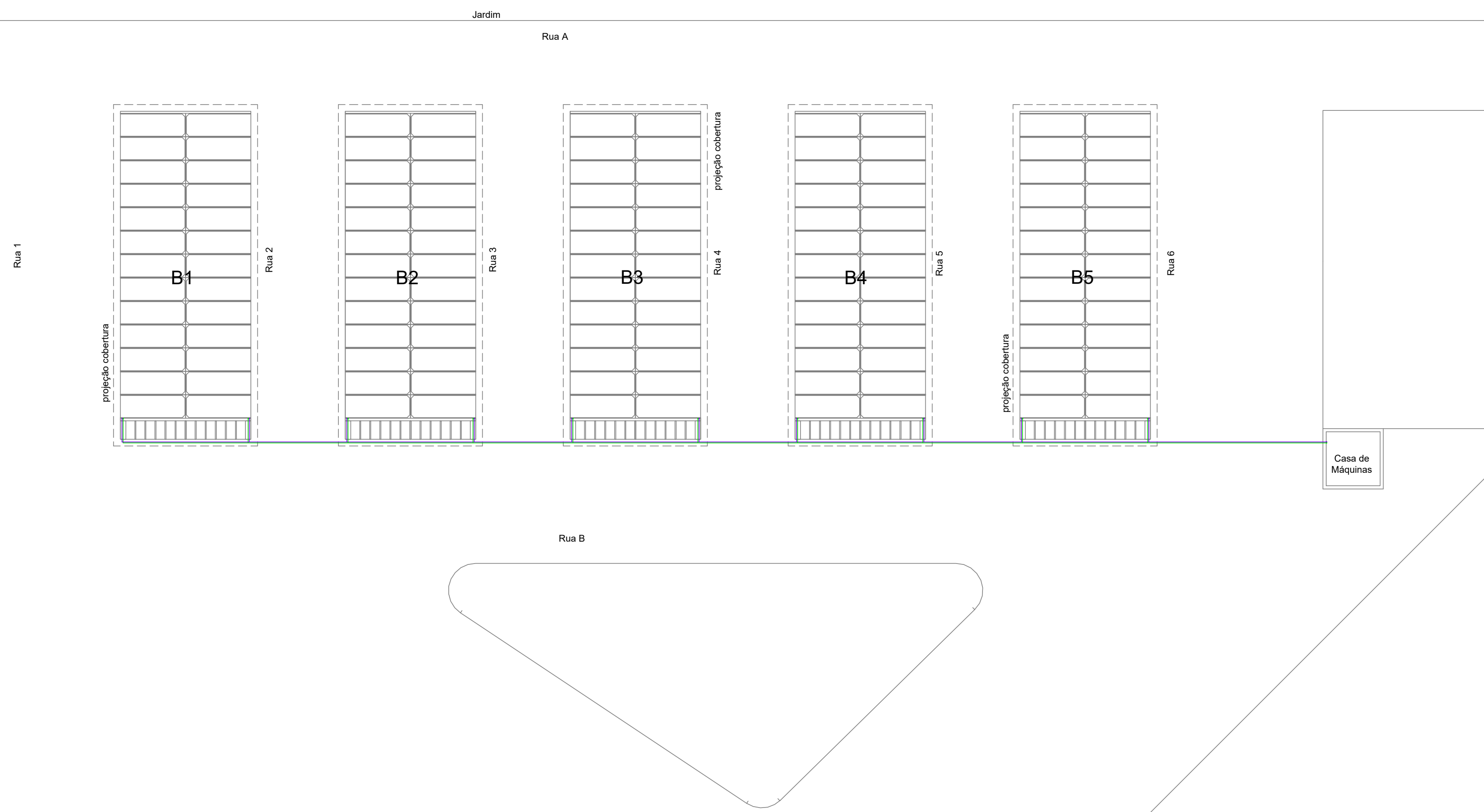
01 IMPLANTAÇÃO-VENTILAÇÃO GAVETAS ESCALA 1:125
