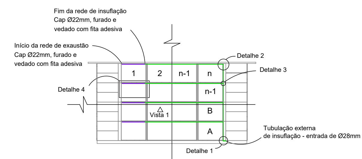
03 CORTE AA ESCALA 1:75
