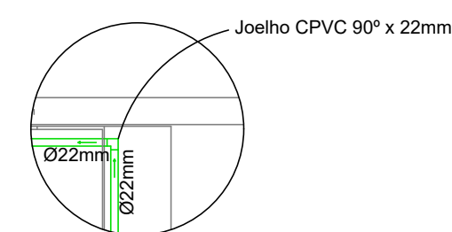
05 DETALHE 2 ESCALA 1:20
