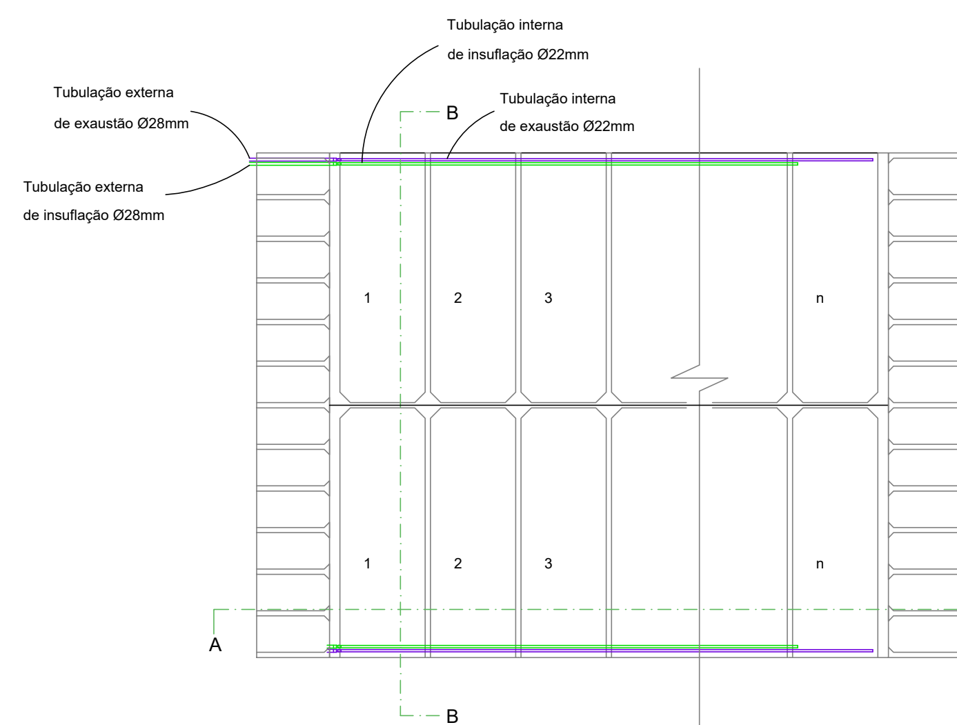
07 LIGAÇÃO GAVETAS ESCALA 1:50
