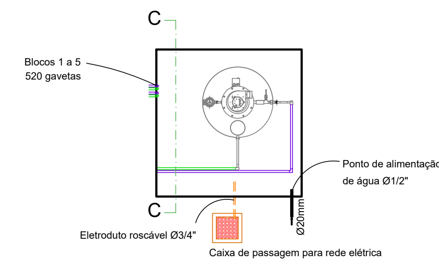
12 LIGAÇÃO CASA DE MÁQUINAS ESCALA 1:50
