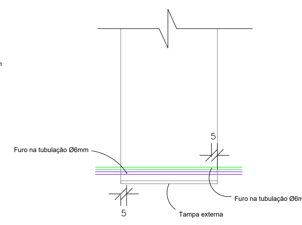
09 VISTA 1 ESCALA 1:20
