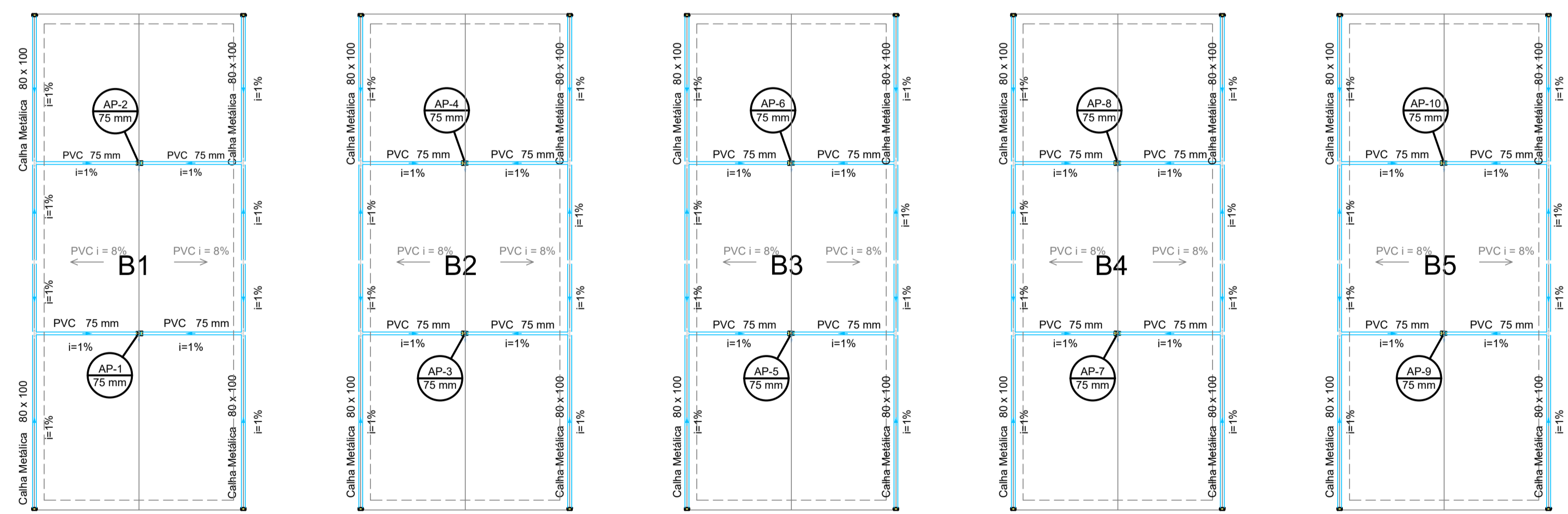
02 PLANTA COBERTURA - DRENAGEM PLUVIAL ESCALA 1:100
