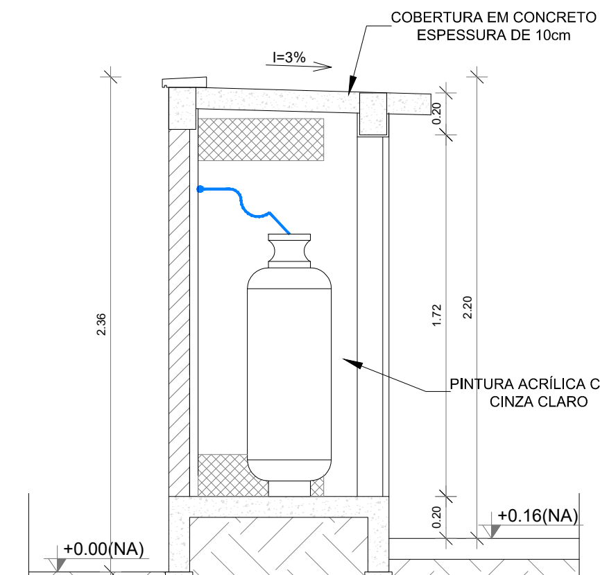
5 CORTE AA 1/25
