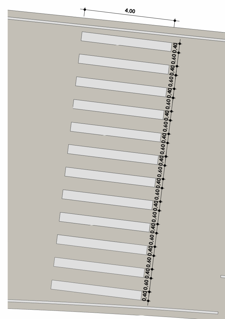
DETALHE DA FAIXA DE PEDESTRE ESC: 1 : 100
