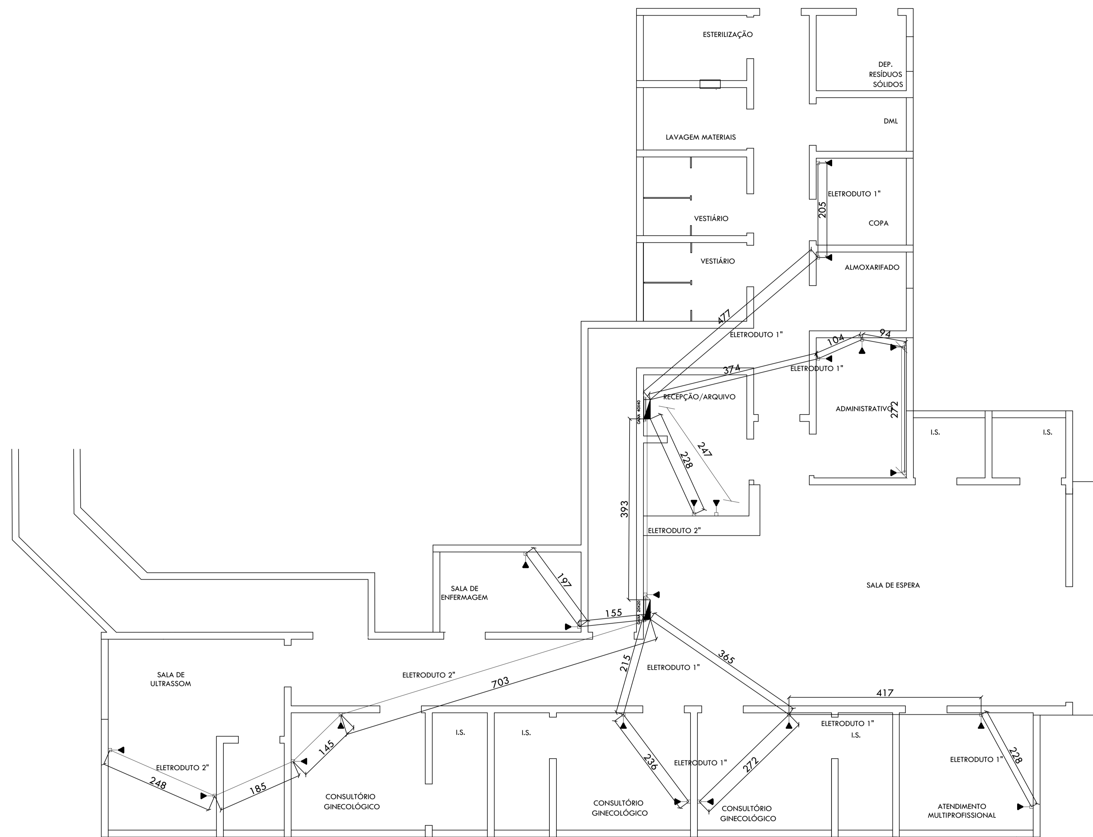
PLANTA DE REDE ESCALA 1:50
