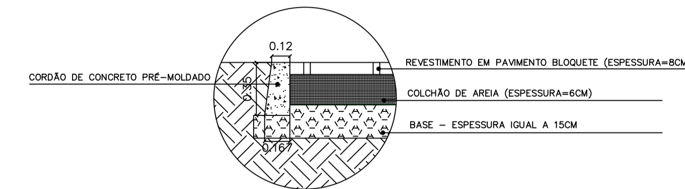
07 DETALHE MEIO FIO PRÉ MOLDADO ESCALA 1:20
