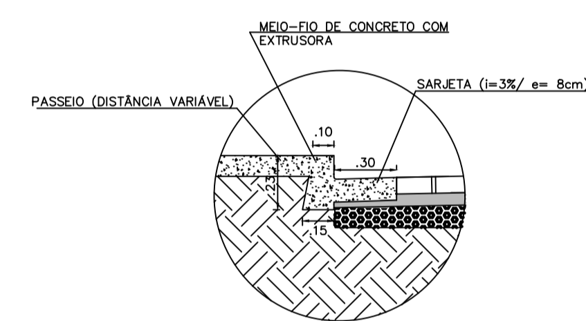
08 DETALHE SARJETA ESCALA 1:20
