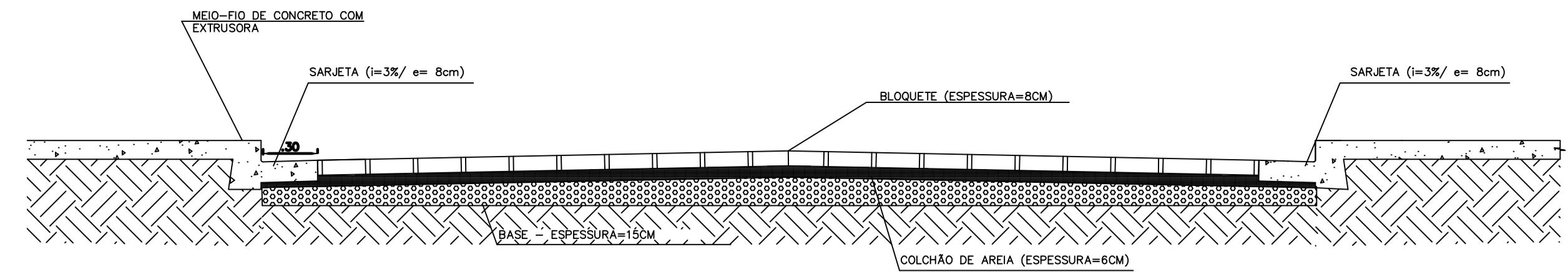
05 DETALHE DO CALÇAMENTO COM BLOCOS SEXTAVADOS ESCALA 1:20
