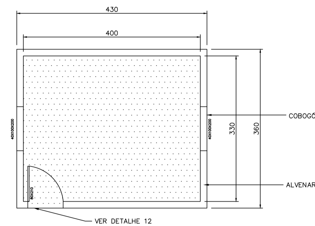
09 CASA DE BOMBA ESCALA 1:50
