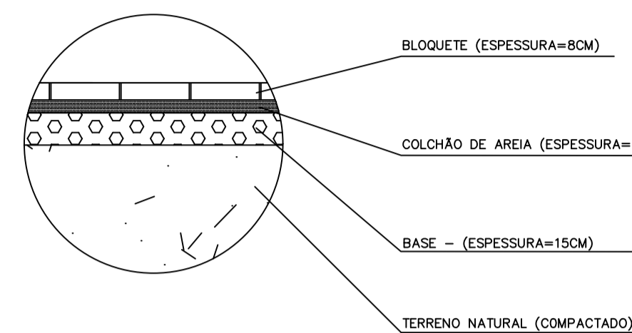
06 CAMADAS DO CALÇAMENTO ESCALA 1:20
