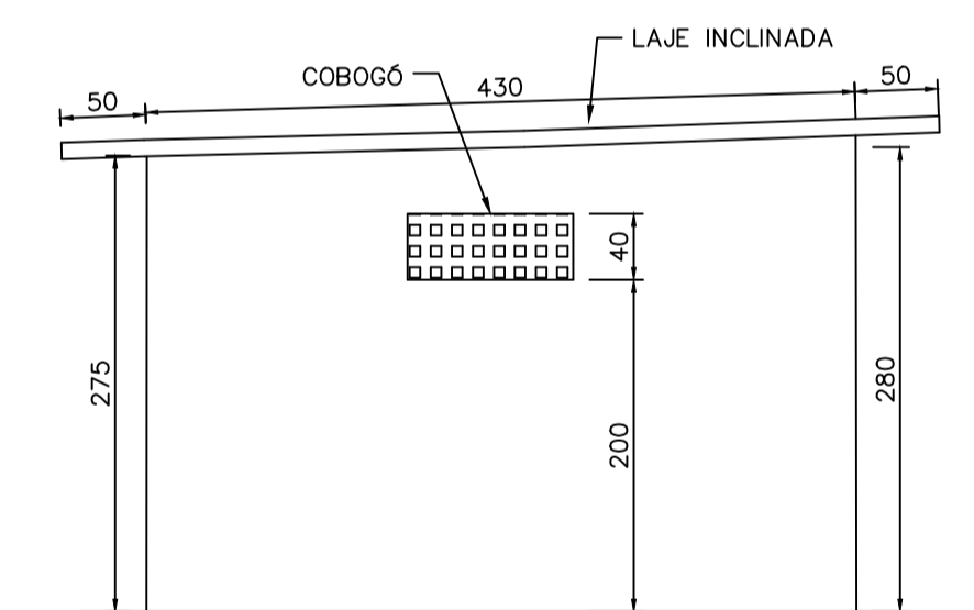
10 CASA DE BOMBA VISTA LATERAL ESCALA 1:50
