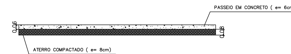
15 CORTE TRANSVERSAL PASSEIO ESCALA 1:20
