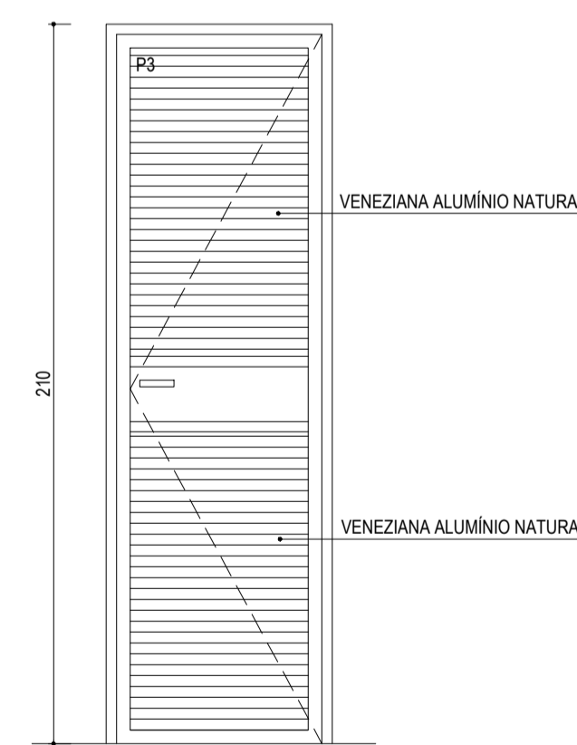
P3 - ELEVACÃO INTERNA ESCALA 1:20
