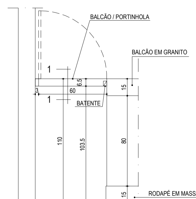
VISTA 3 ESCALA 1:20
