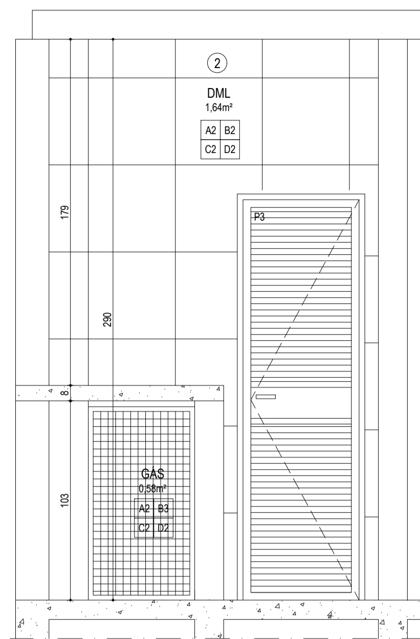
SEÇÃO 1.1 ESCALA 1:20
