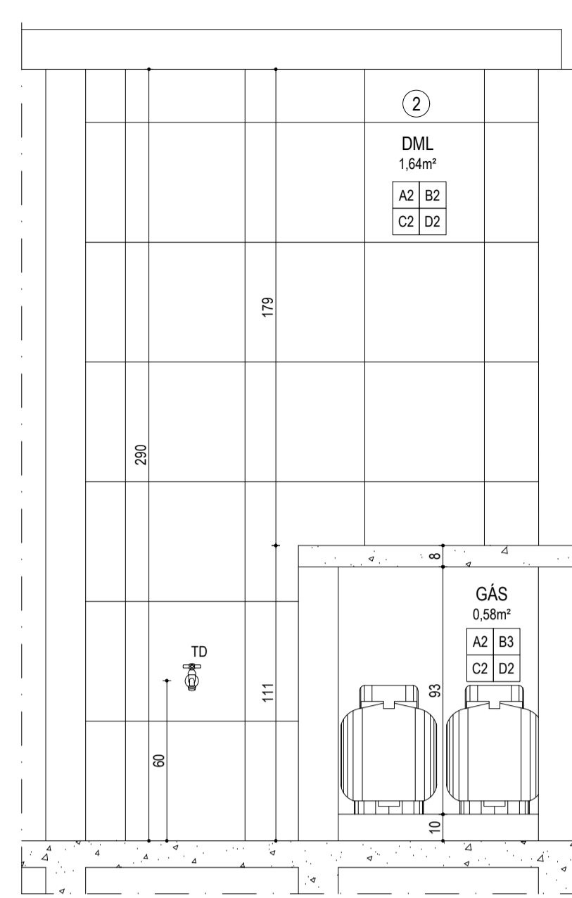
SEÇÃO 2.2 ESCALA 1:20
