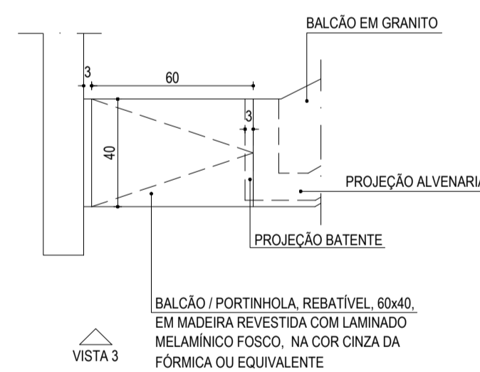
PORTINHOLA ACESSO RESTRITO ATENCIMENTO - PLANTA ESCALA 1:20
