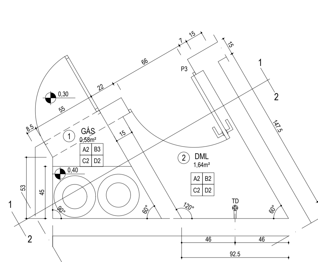
AMPLIAÇÃO - GÁS / DML - PLANTA A03 ESCALA 1:20 01/05
