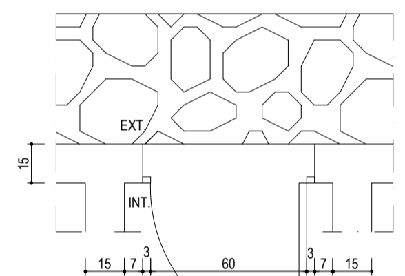
P3 - PLANTA ESCALA 1:20
