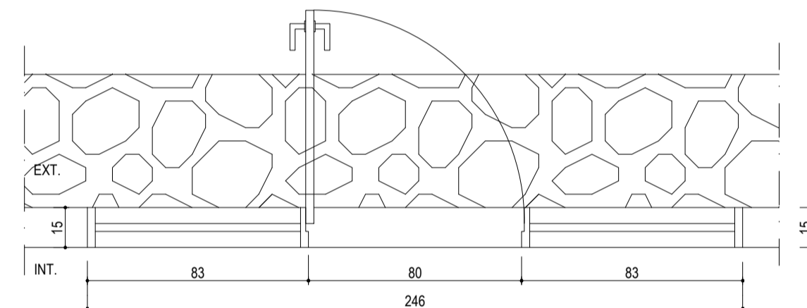
J2 / P2 - PLANTA ESCALA 1:20
