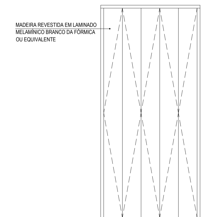
P4 - ELEVACÃO VARANDA ESCALA 1:20
