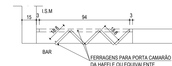
P4 - PLANTA ESCALA 1:20
