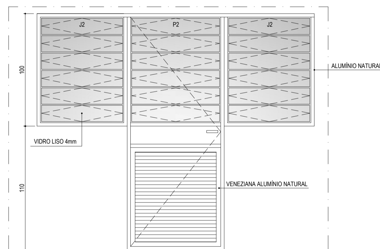
J2 / P2 - ELEVACÃO INTERNA ESCALA 1:20
