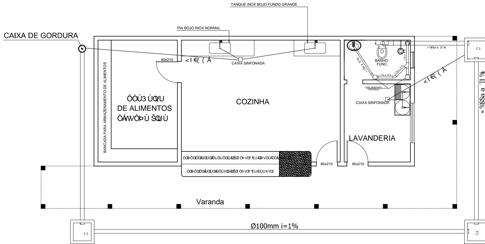
Planta Baixa Escala: 1/75
