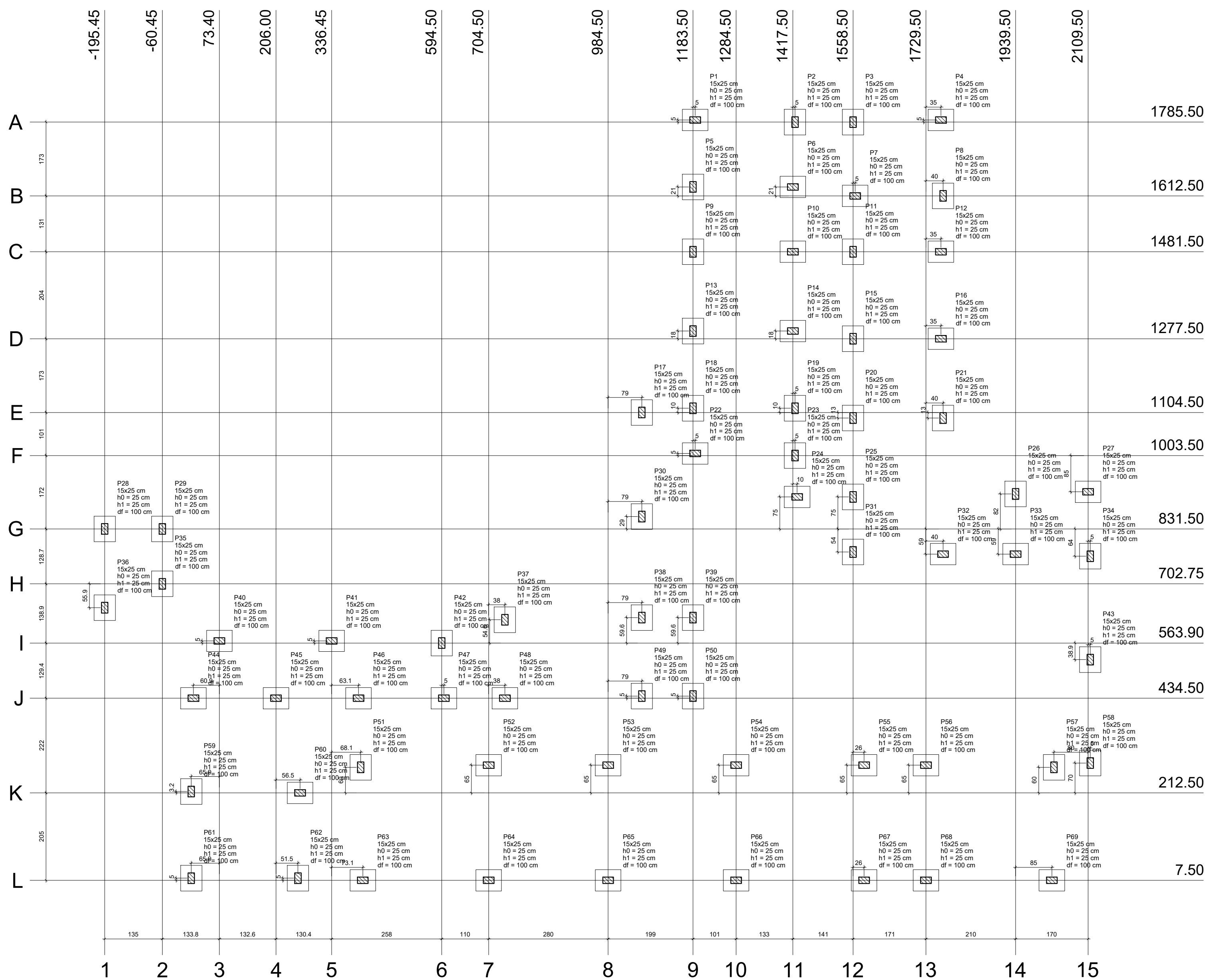
Planta de localização escala 1:50
