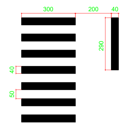
DETALHE 1 FAIXA DE PEDESTRES RUAS LARGURA 7 m 9,56 m 2
