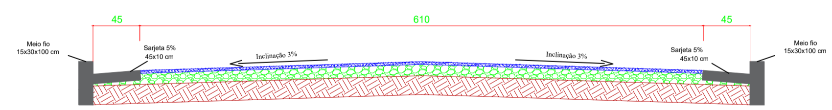
CORTE TRANSVERSAL SI ESCALA
