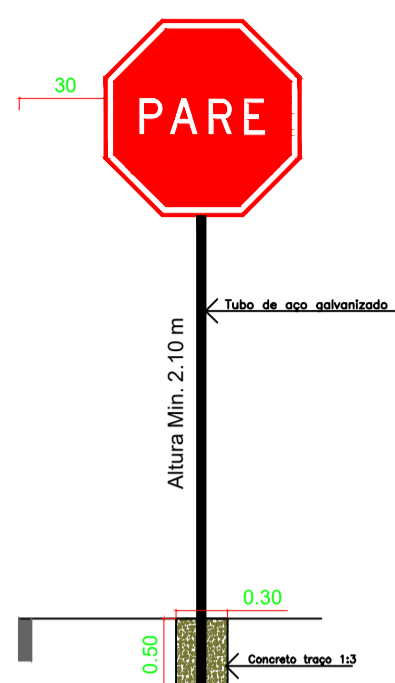
DETALHE 2 PLACA DE SINALIZAÇÃO
