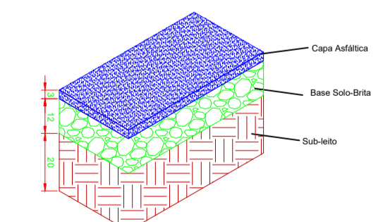
CAMADAS PAVIMENTO SI ESCALA
