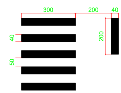
DETALHE 1 FAIXA DE PEDESTRES RUAS LARGURA 5 m 6,08 m 2
