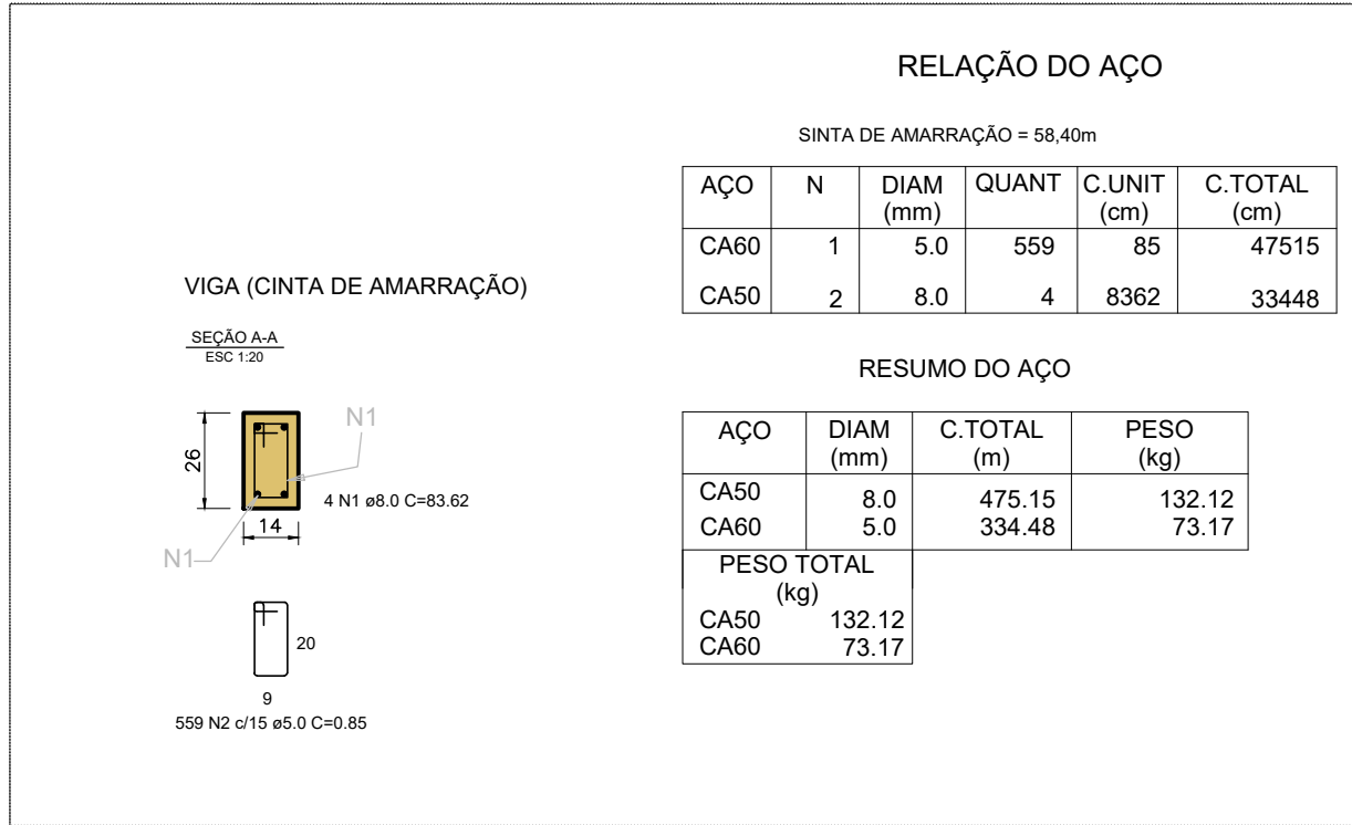
9 DETALHE - CINTA DE AMARRAÇÃO DO MURO ESCALA 1:25
