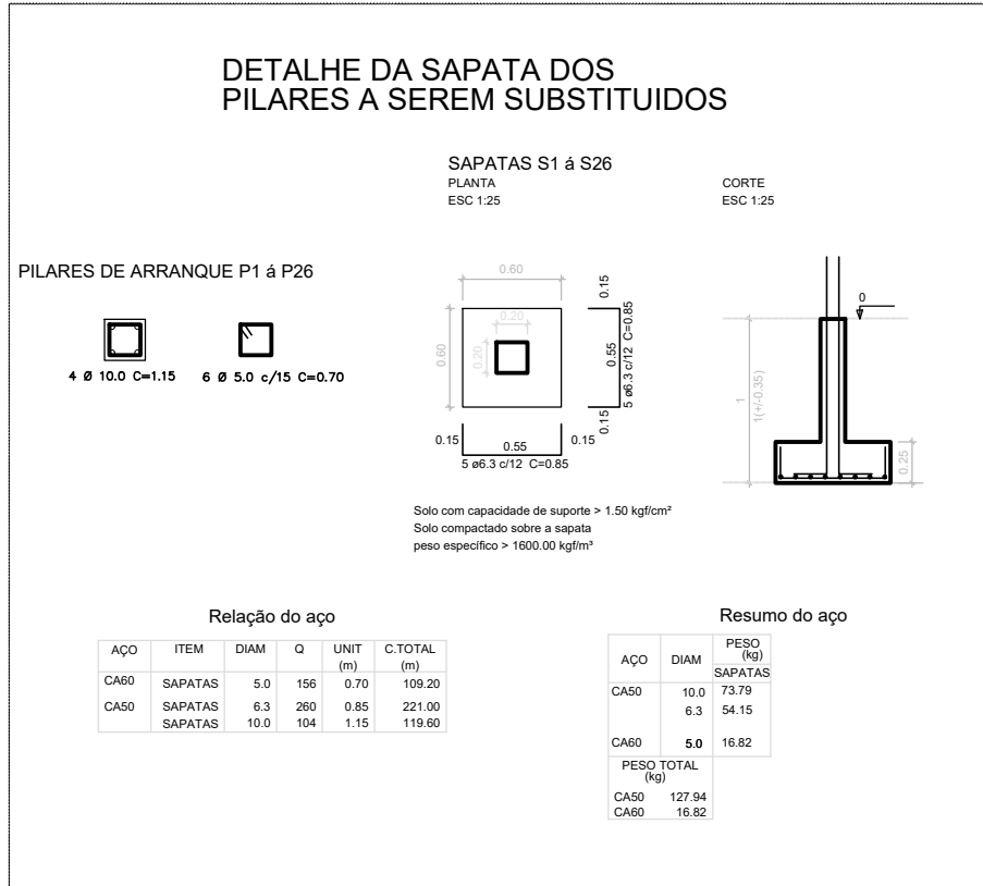
10 DETALHE - SAPATA DOS PILARES SUBSTITUIDOS ESCALA 1:25
