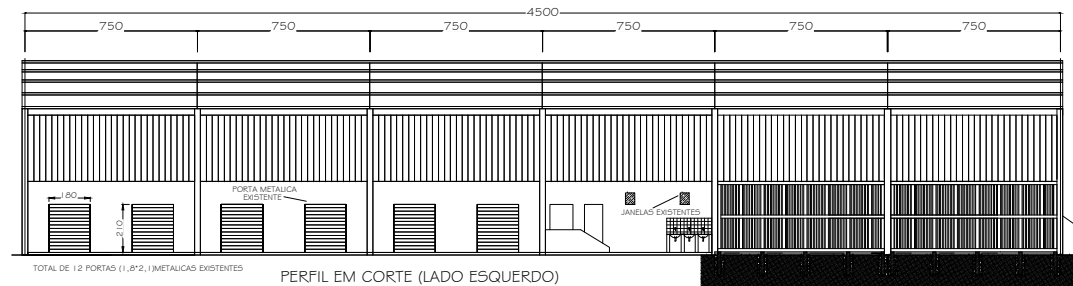
PERFIL EM CORTE (LADO ESQUERDO)
