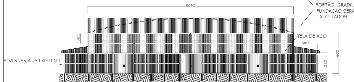
FACHADA POSTERIOR.
