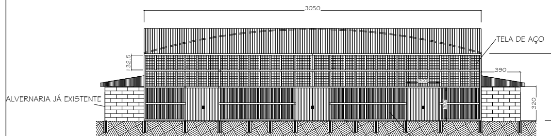
FACHADA PRINCIPAL.
