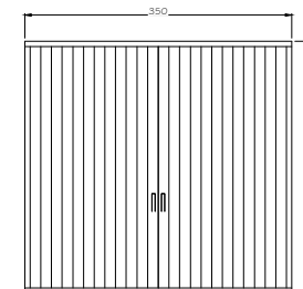
DETALHE (PORTÕES).
