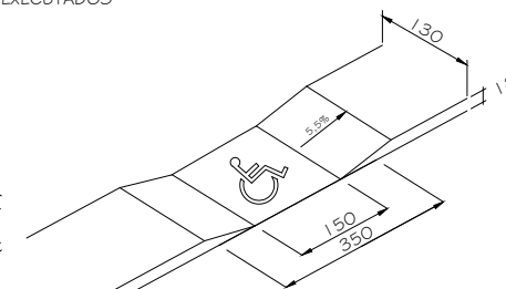
ISOMÉTRICO DO ACESSO A DEFICIENTES INCLINAÇÃO DE 5,5%( CALÇADA, FRENTE E FUNDOS) POSICIONAMENTO NA PLANTA (PRANCHA 2)
