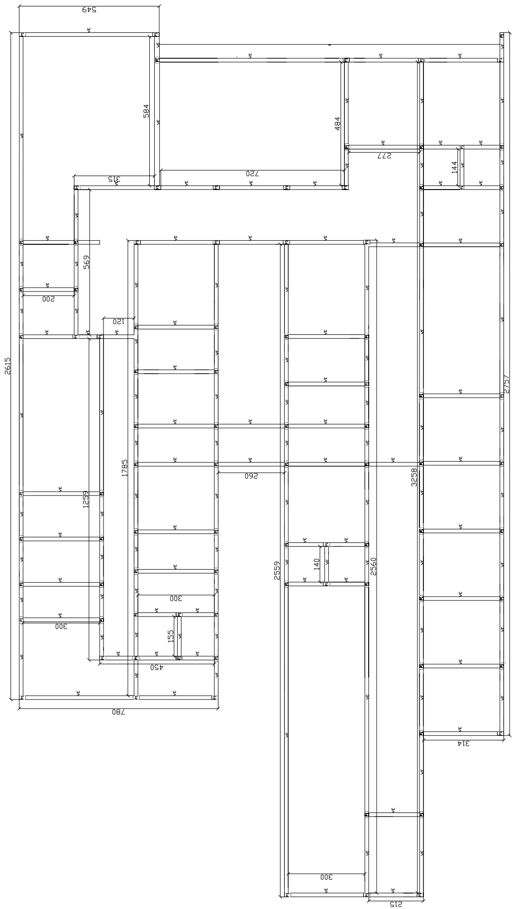
PLANTA BAIXA DE FORMA esc 1:100
