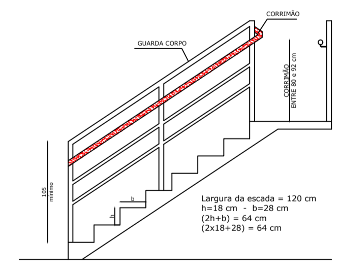
DETALHE GUARDA CORPO E CORRIMÃO DA ESCADA
