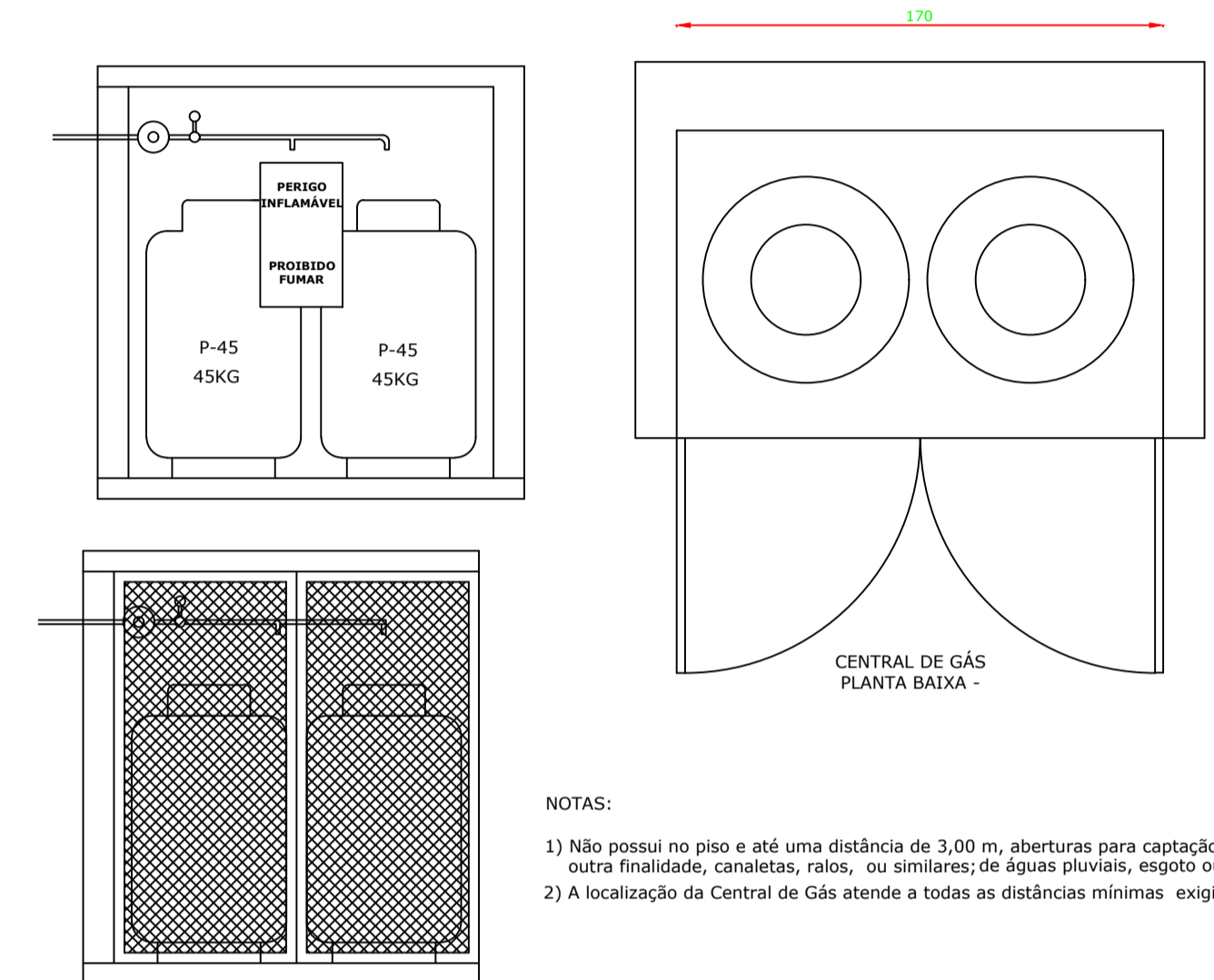
CENTRAL DE GÁS VISTA FRONTAL
