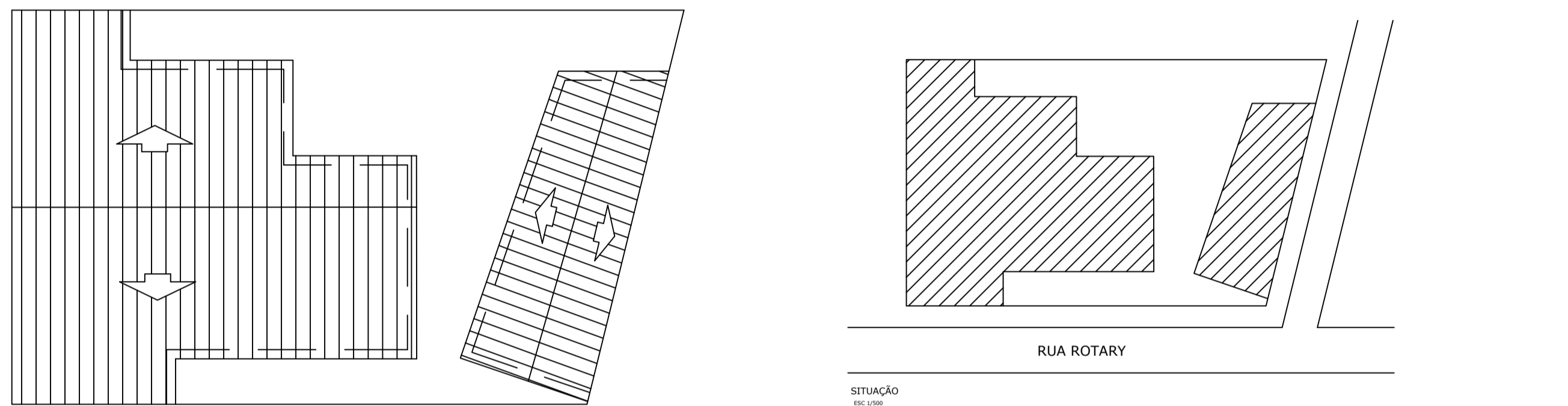
COBERTURA ESC 1/200
