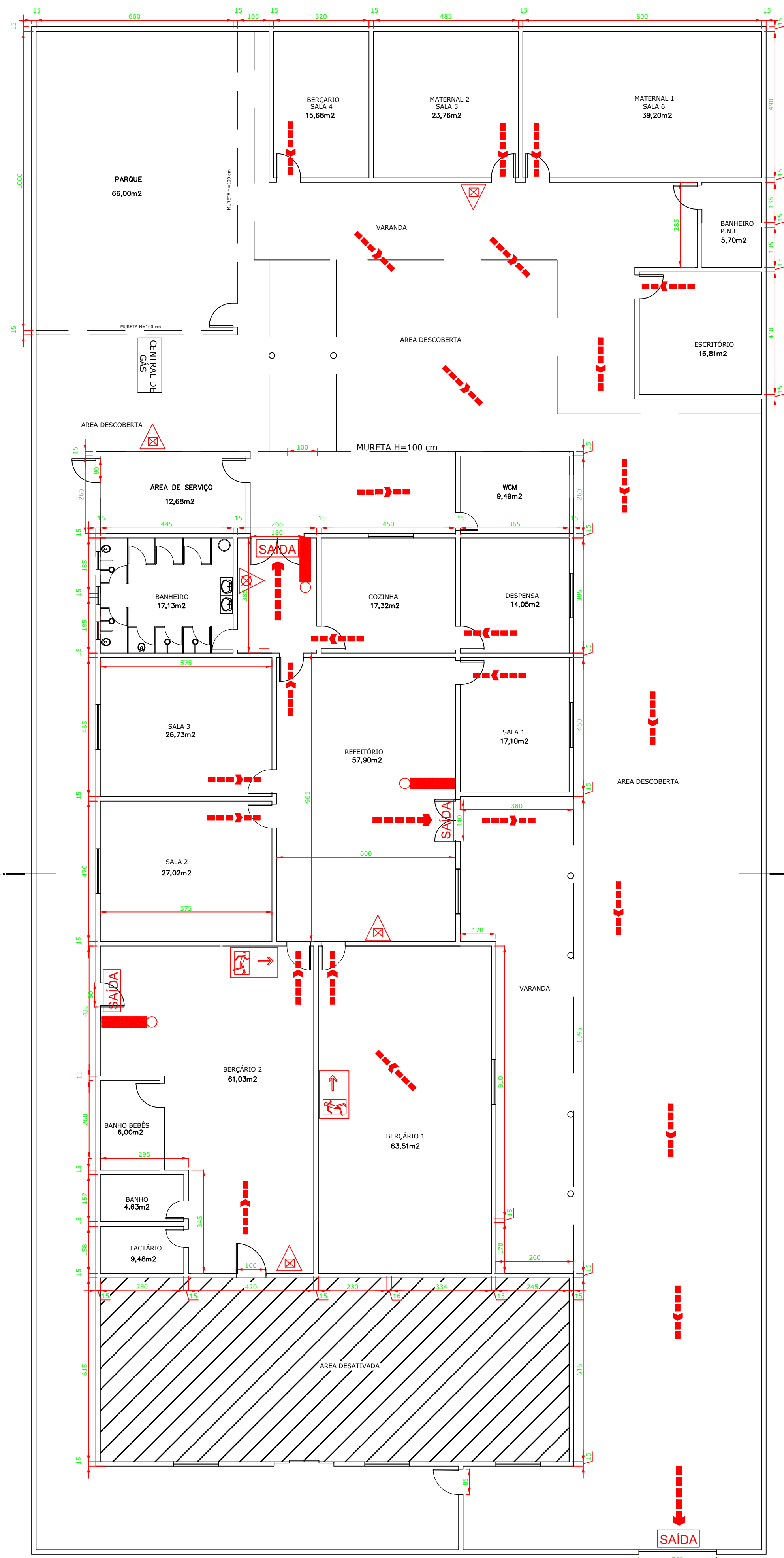
PLANTA BAIXA ESC 1/100
