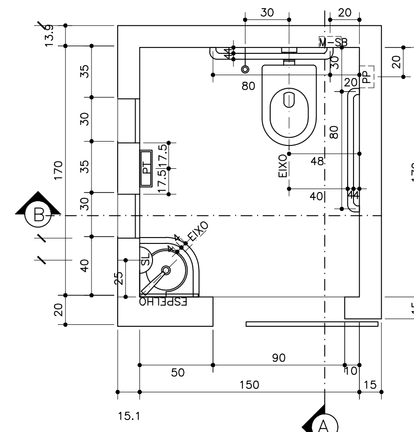
DETALHE BANHEIRO ESPECIAL esc 1:20
