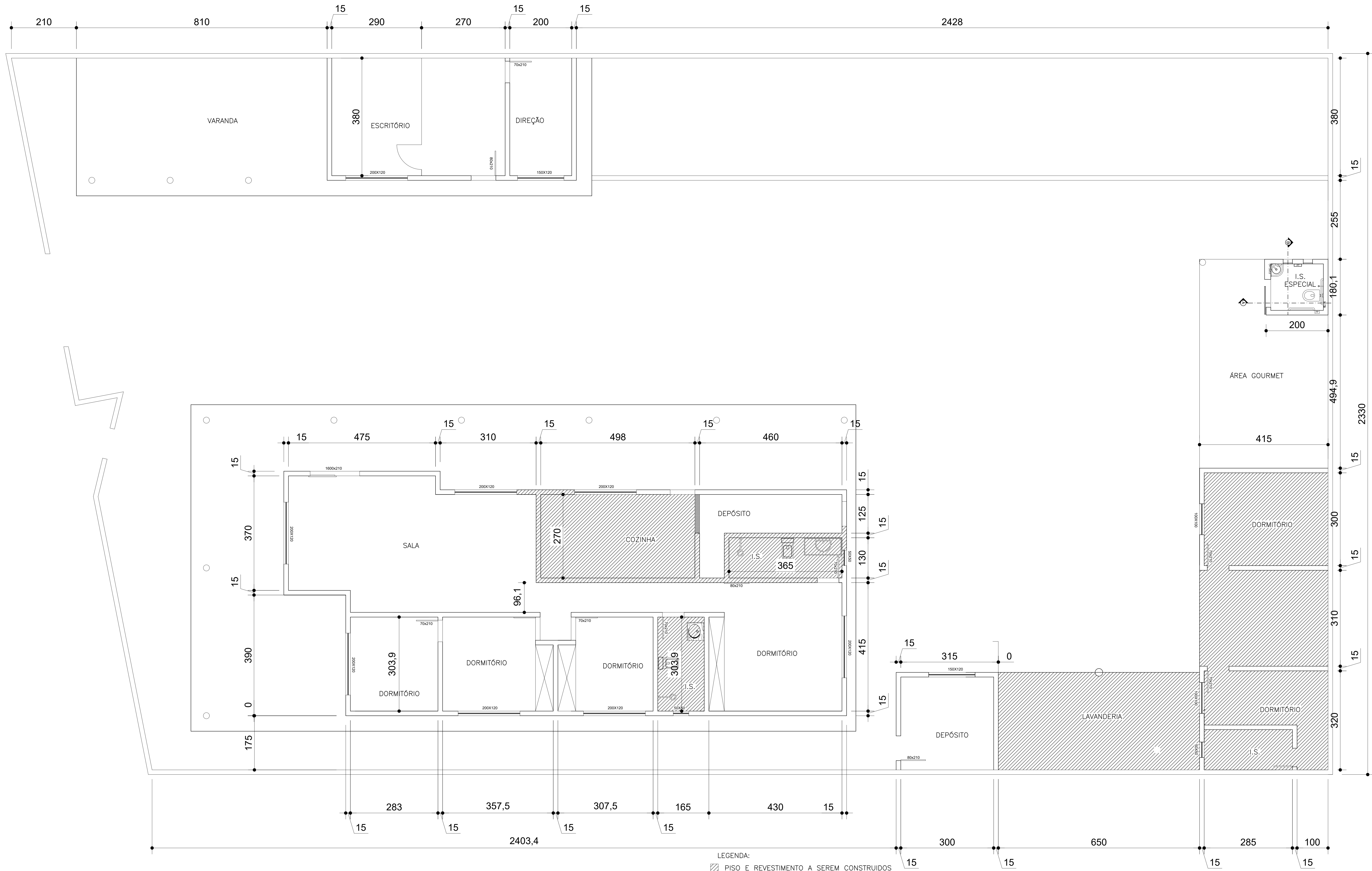
PLANTA esc 1:100
