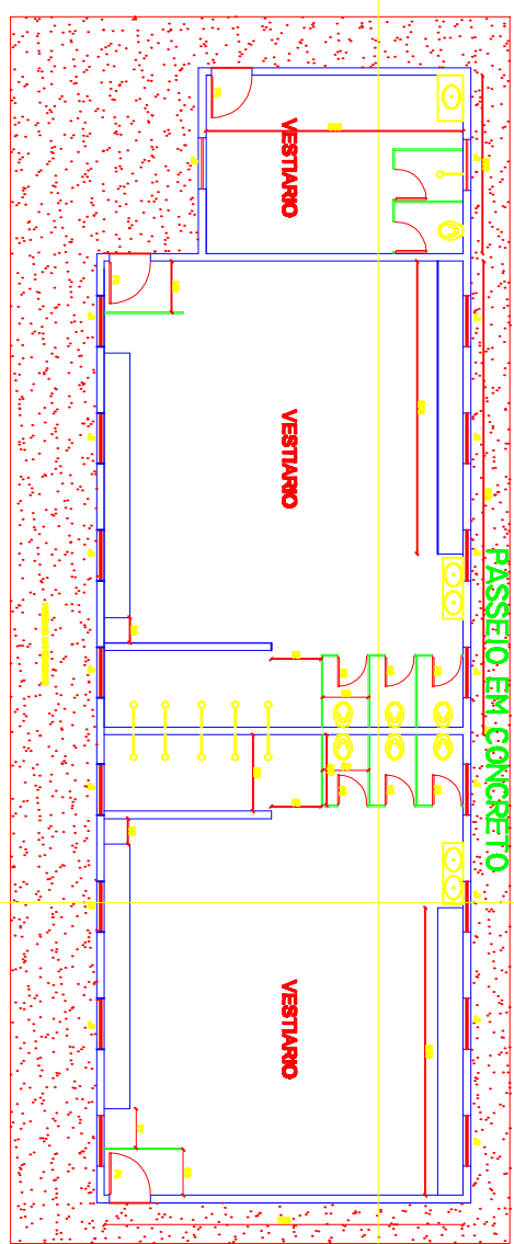
PLANTA BAIXA VESTIBULAR ESCALA 1:50
