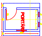
PLANTA BAIXA PORTAL AA ESCALA 1:50
