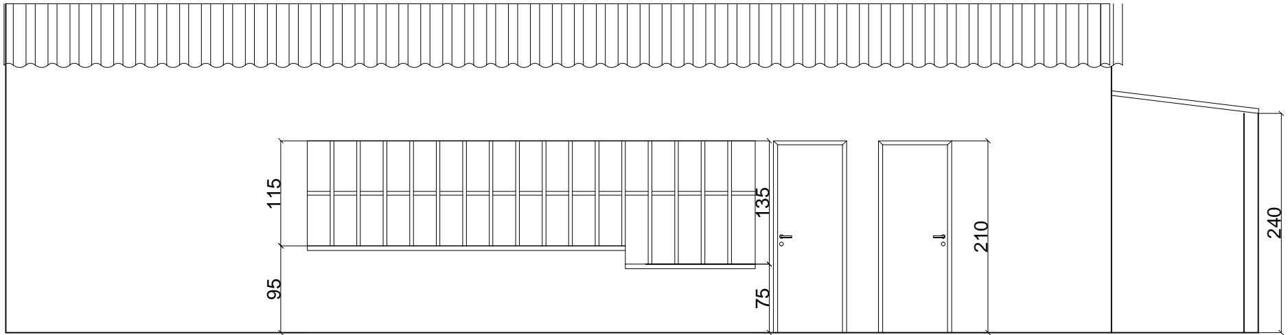
Fachada Escala: 1/50
