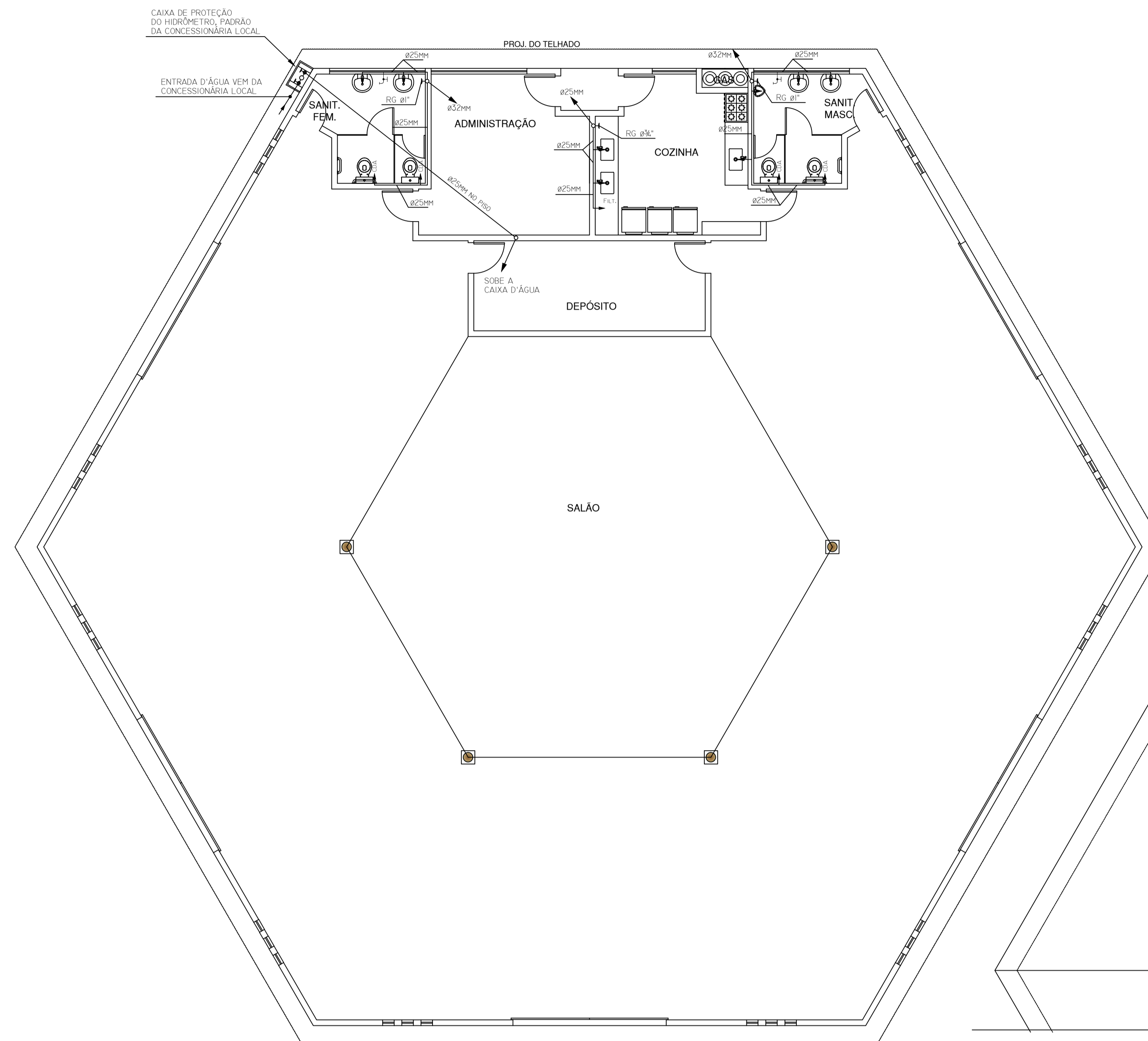
1 PLANTA BAIXA DO TÉRREO ESCALA: 1:75
