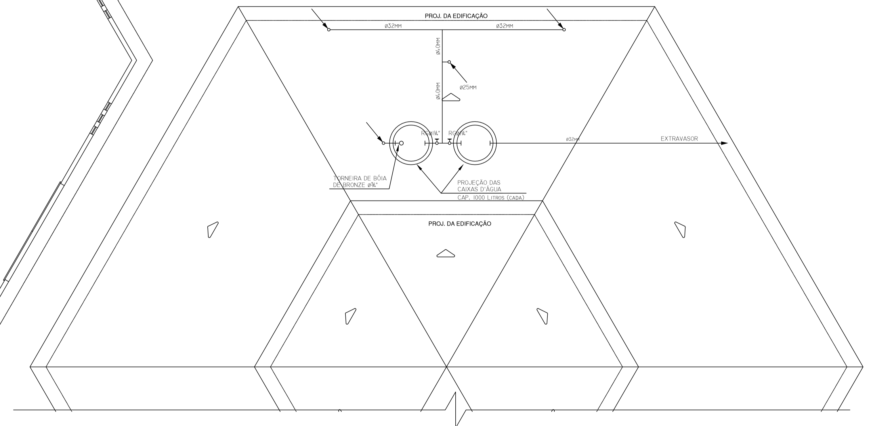
2 PLANTA DE COBERTURA ESCALA: 1:75
