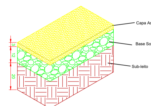
CAMADAS PAVIMENTO
