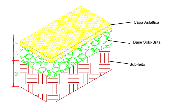
CAMADAS PAVIMENTO S/ ESCALA
