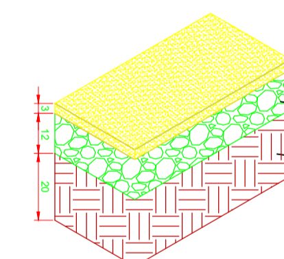
CAMADAS PAVIMENTO S/ ESCALA
