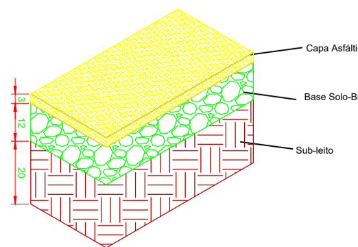
CAMADAS PAVIMENTO SI ESCALA
