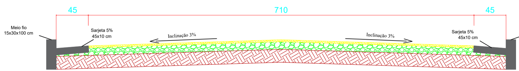
CORTE TRANSVERSAL SI ESCALA
