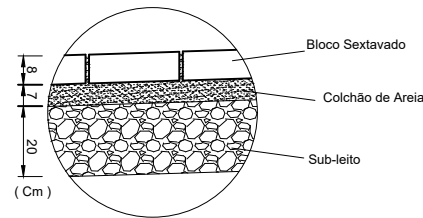
CORTE TRANSVERSAL S/ ESCALA
